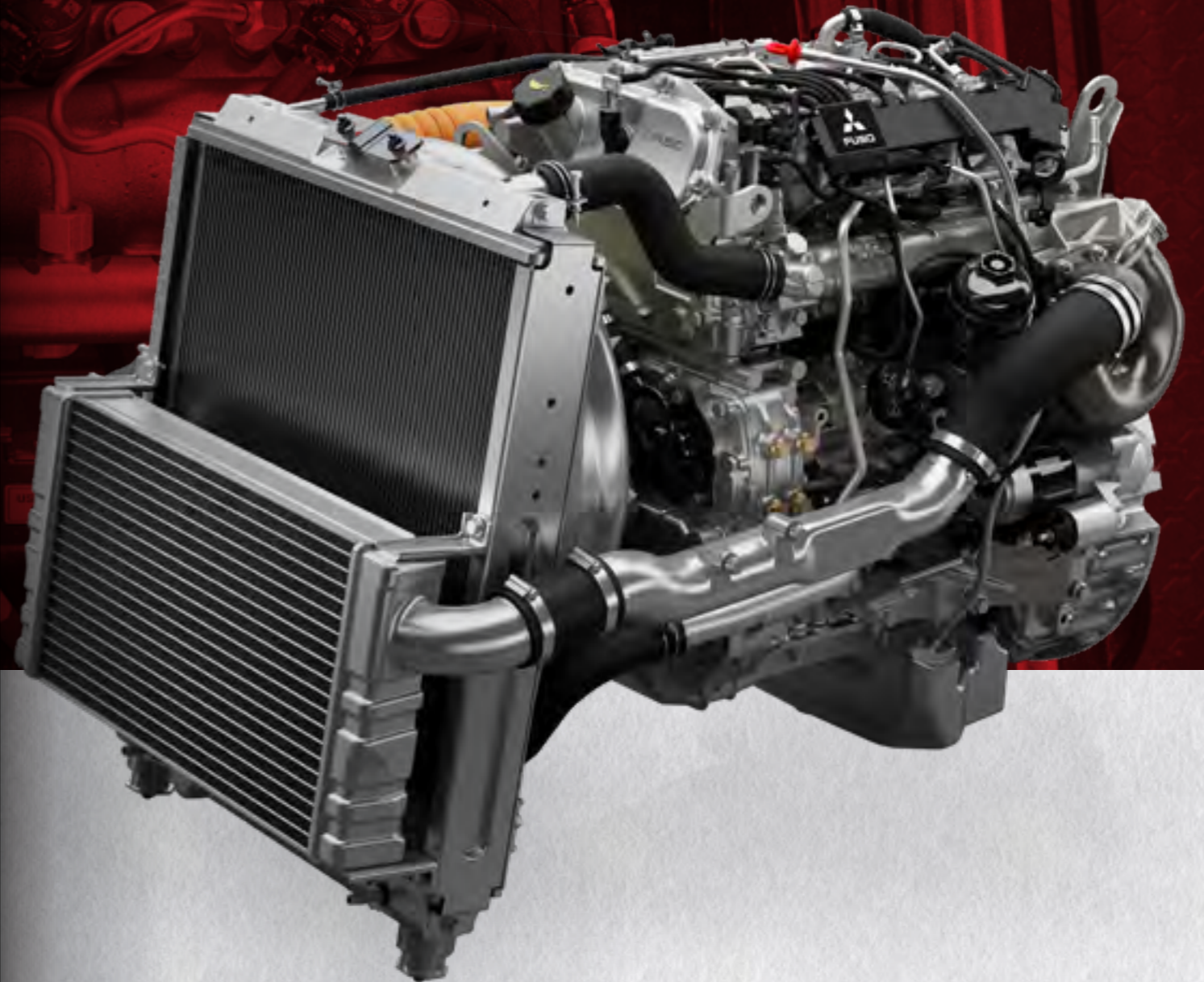
Fuso 4P-10 T6
