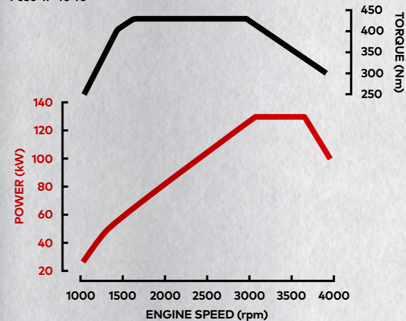
Fuso 4P-10 T6
